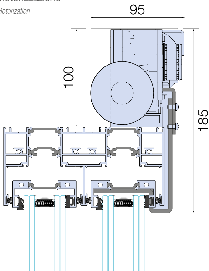
schema applicazione superiore motorizzazione
