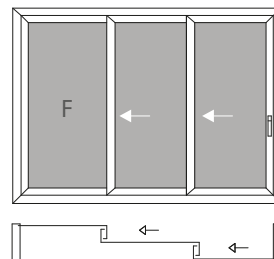
6A 3 vie - 2 ante+fisso 3 rail-2 sash+fixed
