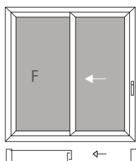
3A 2 vie - 1 anta+fisso 2 rail-1 sash+fixed
