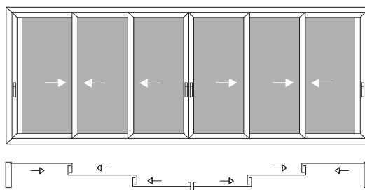
9A 3 vie - 6 ante 3 rail-6 sash
