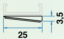
Sottoguida inclinata 7° per compensazione soglia (opzionale)
