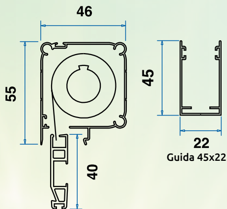
Cassonetto con tubo, rete e barra maniglia
