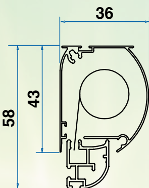
Cassonetto da 36 mm
