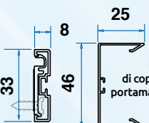
Profilo di riscontro ridotto (opzionale)
