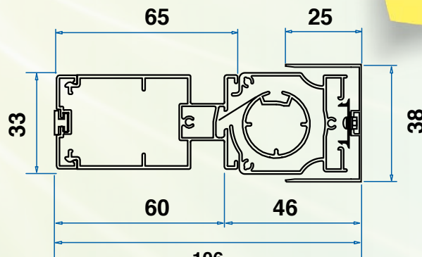
Pacchetto Rete con barramaniglia Maxxy
