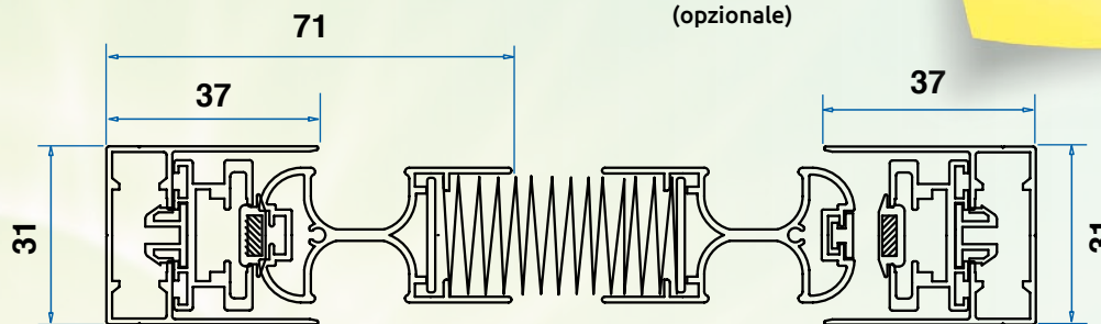
Profilo di riscontro
