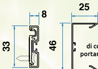
Profilo di riscontro ridotto (opzionale)
