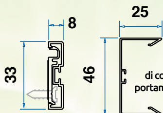
Profilo di riscontro ridotto (opzionale)
