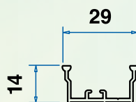
Barra di riscontro (solo per anta singola)
