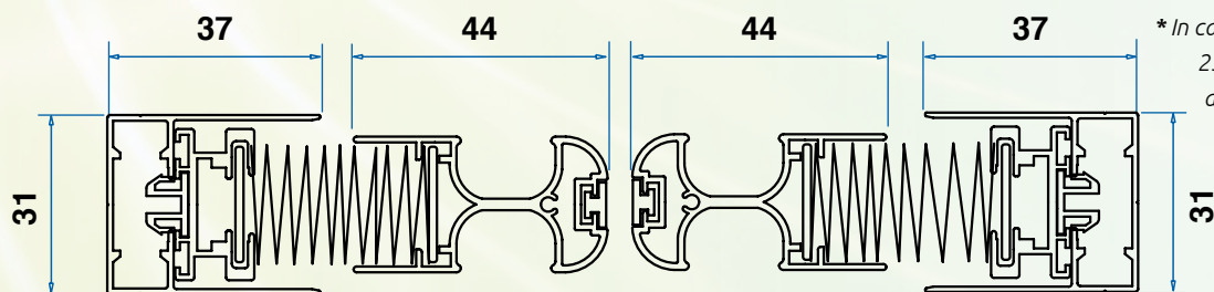
Profilo di riscontro
