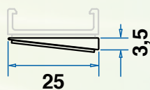
Sottoguida inclinata 7° per compensazione soglia (opzionale)
