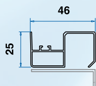
Barra di riscontro*
