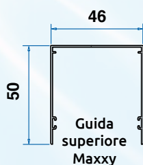
Guida superiore Maxxy
