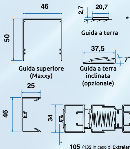
Barra di riscontro da incasso (Maxxy)
